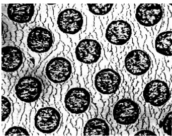
Abriebbild einer verschromten Ballardhaut nach 2 Mill. Umdrehungen Schuppenbildung zerstört Vergr. 160:1
