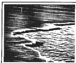
REM-Aufnahme der durch Schuppenbildung zerstörten Chromoberfläche Vergr. 8000:1
